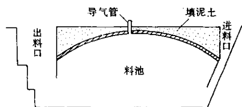
图2 船形沼气池示意图
