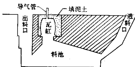
图1 瓦缸沼气池示意图
