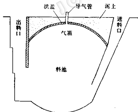
图3 锅形沼气池示意图
