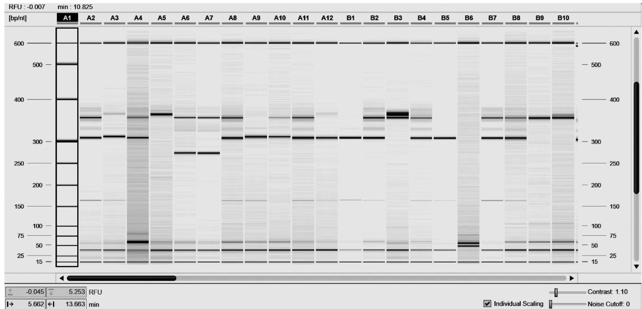
图 3. 引物 SSR 96 部分 PCR 扩增结果毛细管电泳检测图
