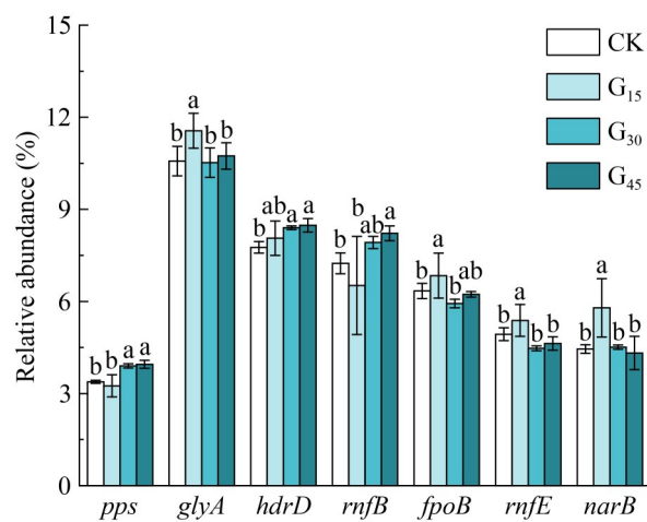
图5 不同石膏用量条件下苏打盐碱稻田土壤甲烷氧化功能基因的相对丰度。不同小写字母表示处理间差异显著( P<0.05 )。
