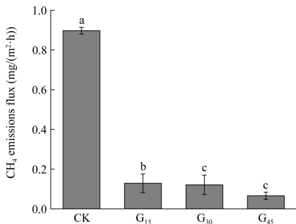
图1 不同石膏用量条件下苏打盐碱稻田CH 4 排放通量。不同小写字母表示处理间差异显著( P<0.05 )。 Figure 1 CH 4 emission fluxes from saline-sodic paddy fields under different gypsum application rates. Different lowercase letters indicate significant differences ( P<0.05 ).
