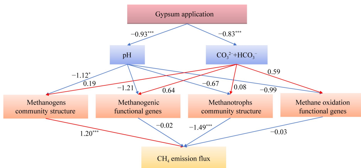
图7 石膏改良剂影响苏打盐碱稻田CH 4 排放通量的PLS路径分析。箭头旁边的数字表示路径系数。红线表示正向影响，蓝线表示负向影响。显著性水平用*表示 P<0.05 ，***表示 P<0.001 。
